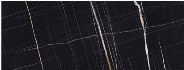
3115/К ОБСИДИАН ЛАБРАДОР
